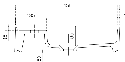
Sezione Section Sección Section
